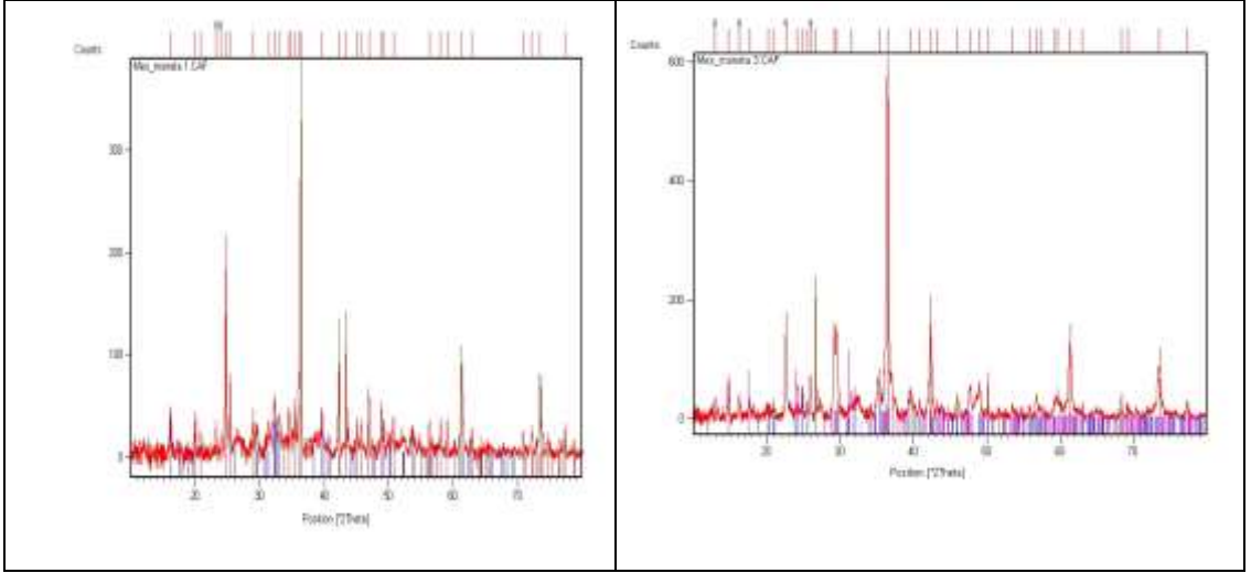
شكل رقم (١٢) راديو غرام للقطعة رقم (01) (Radio gramme RX (Cerussite .Cuprite .Copper . .Chloride .Hydroxide )
